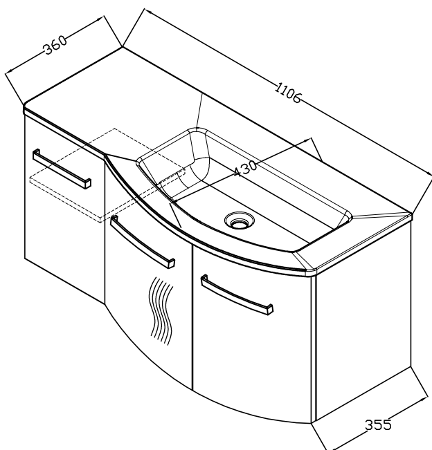
OUE 110 D WH OUE 110 D CAST.GRAPH. / WH
