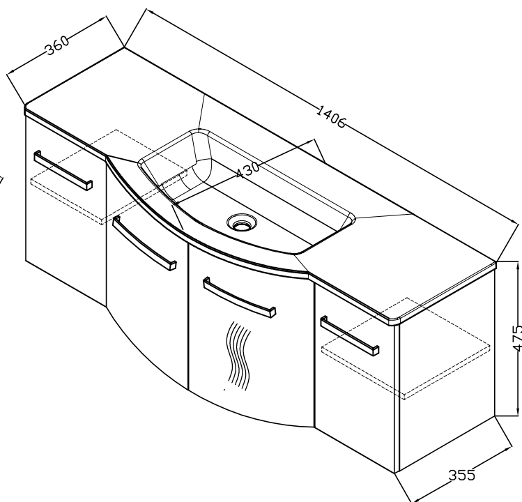
OUE 140 WH OUE 140 CAST.GRAPH. / WH
