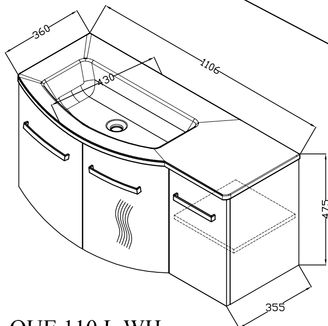
OUE 110 L WH OUE 110 L CAST.GRAPH. / WH
