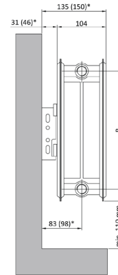
TÍP :22-PKKP
